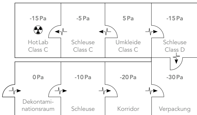
Auszug Druckstufenkonzept Geschoss A
