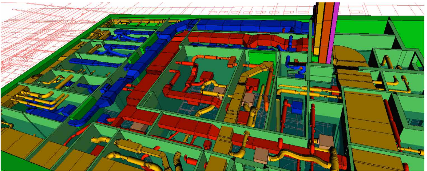
3D-Planauszug Geschoss A
